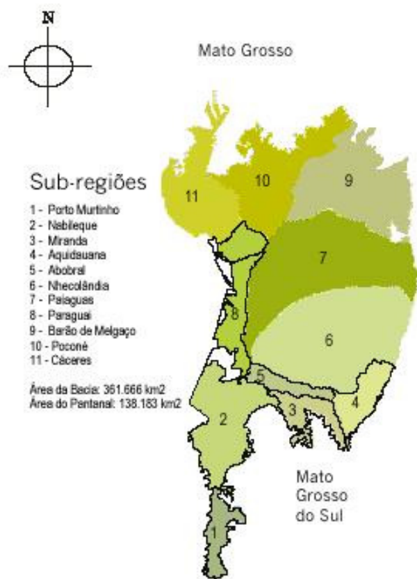
FIGURA 1 - Localização, delimitação e sub-regiões do Pantanal brasileiro (SANTOS et al., 2002 2 ).
