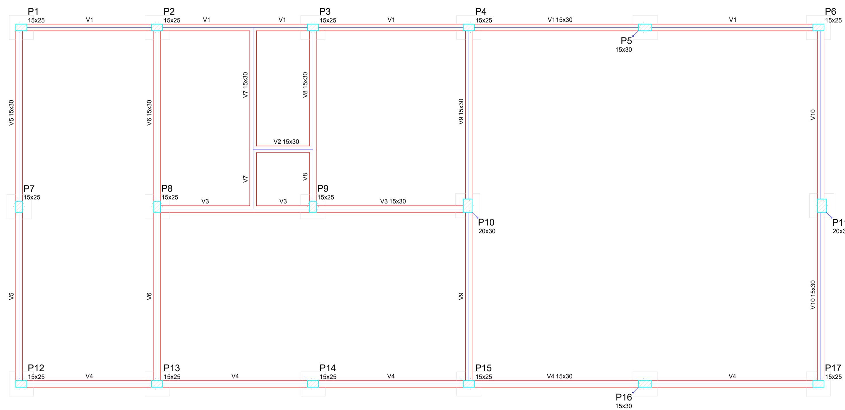
Forma do pavimento fun escala 1:50
